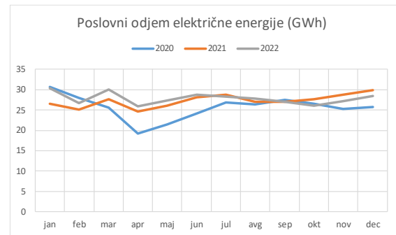
Slika 83: Mesečni poslovni odjem električne energije v Mariboru v obdobju 2020-2022. 142
